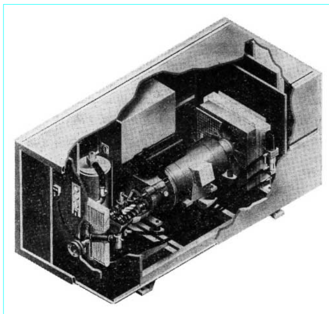
Figure 2 – Éclaté d'un compresseur à vis semi-fixe
