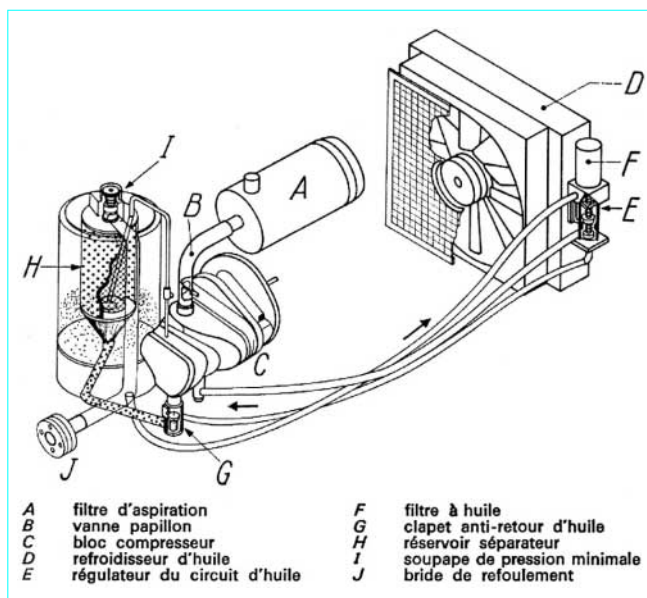
Figure 1 – Schéma de principe d'un compresseur à vis (d'après doc. Sullair)
